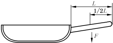
图 7 单柄锅手柄牢固性试验示意图
