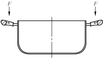
图 6 双柄锅手柄牢固性试验示意图
